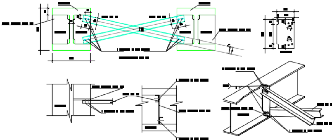
4 3 7 Detalle de Arriostamiento Vigas Metálicas 0 0,4 0,8 1,6m ESCALA 1:10
