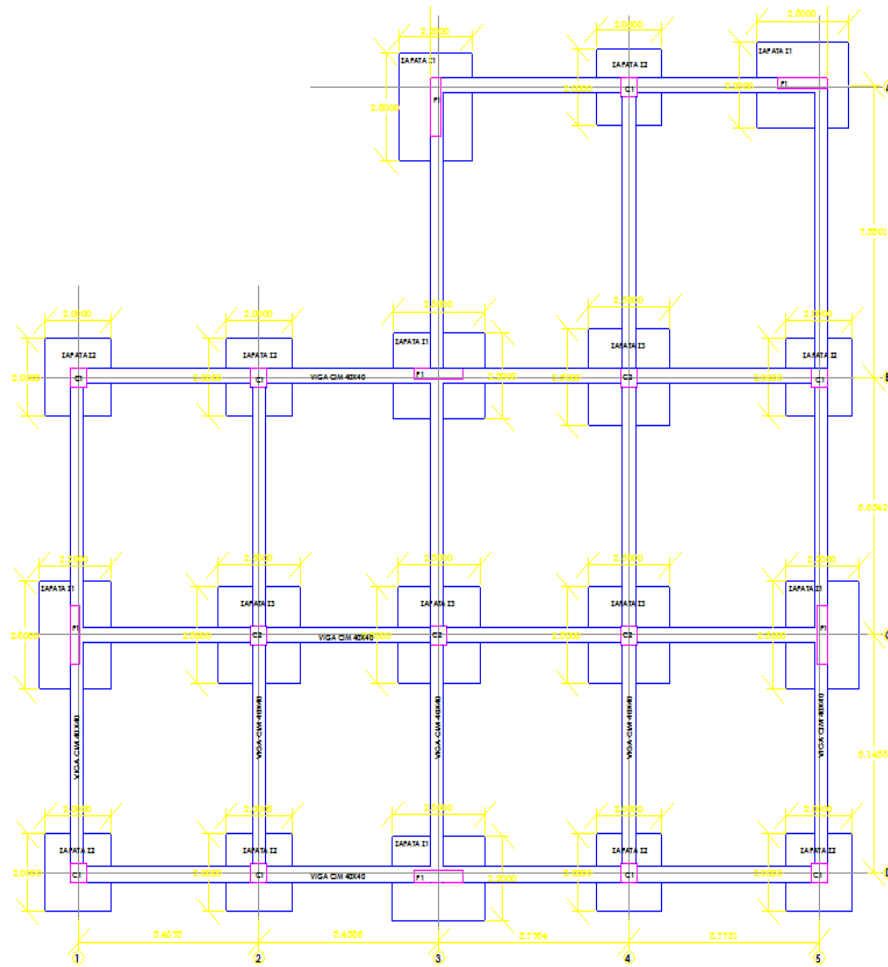
PLANTA DE CIMENTACION LABORATORIO DE DISEÑO MECANICO
