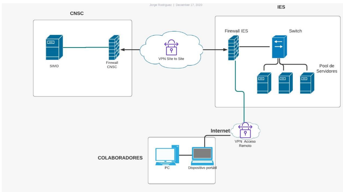
Ilustración 1 Diagrama de conexión.
