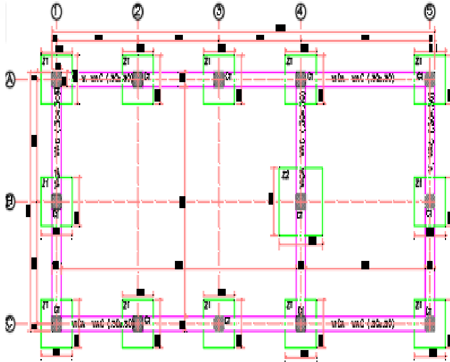
PLANTA CIMENTACION ESC. 1:50
