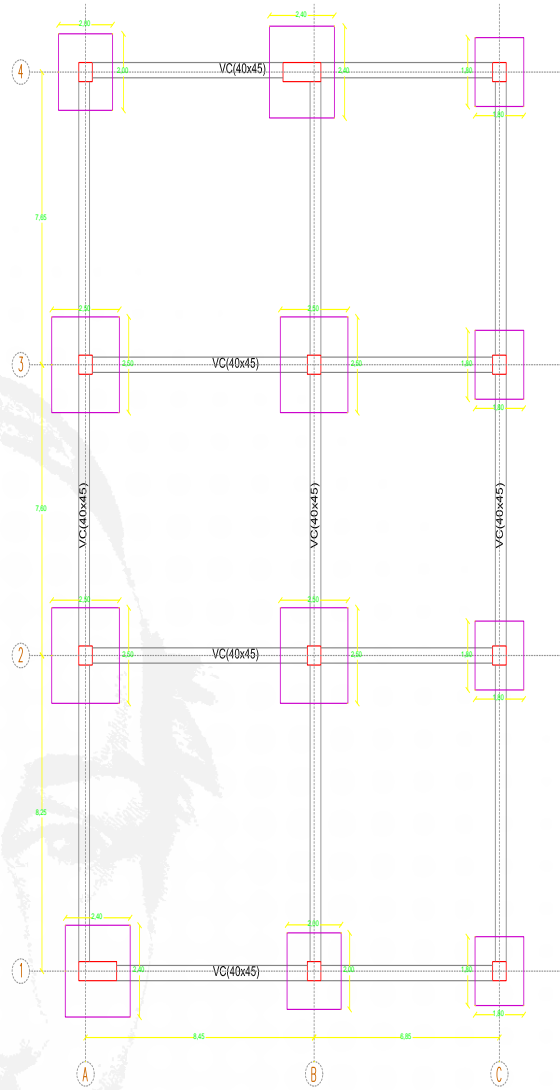
Planta de cimentación
